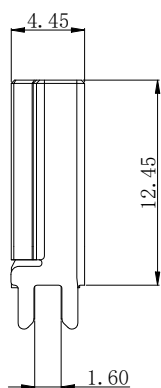
A-A
