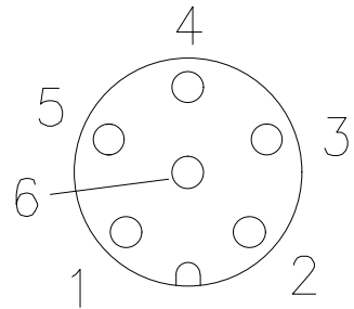
Pin Assingnmnts
